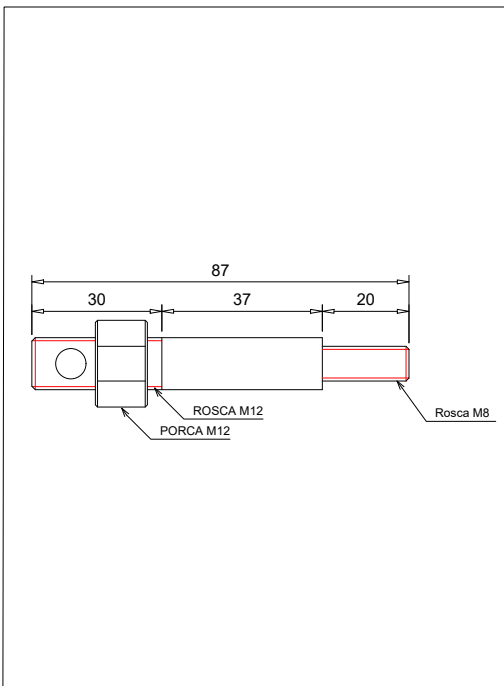
DETALHE "F" Pino de Lacre - Blindado
