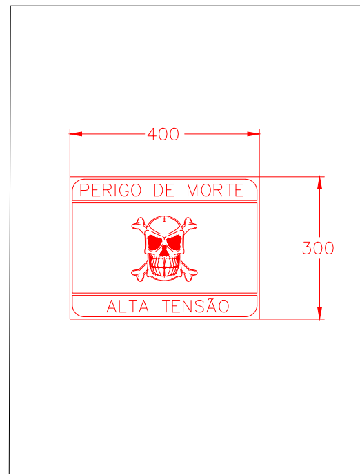
DETALHE "E" Placa de Advertência
