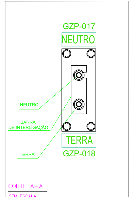
DETALHE "A" EM PERSPECTIVA, INTERLIGAÇÃO FECHADA
