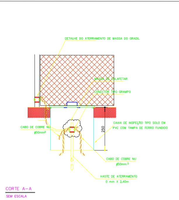
DETALHE "B" Caixa de inspeção e Aterramento da Malha
