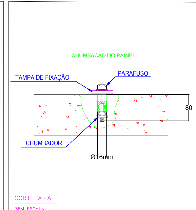
DETALHE "D" Chumbação do Painel
