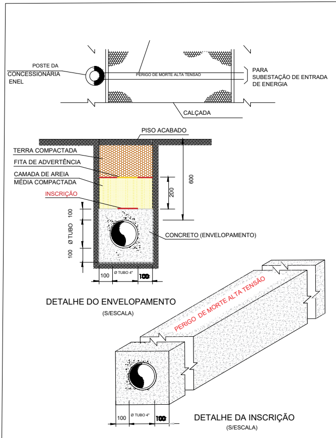
DETALHE "G" Envolvimento
