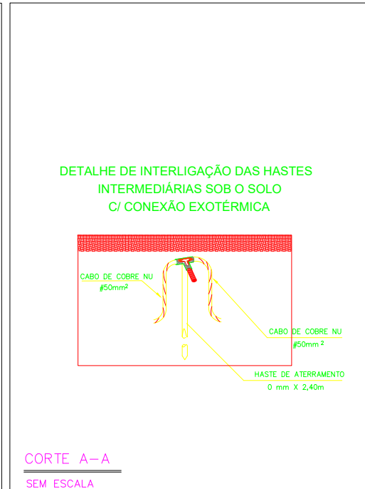
DETALHE "C" Hastes Intermediárias
